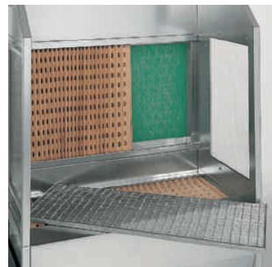
Die Filtermedien, Vor- und Feinfilter, sind bei Bedarf mit wenigen Handgriffen gewechselt.
